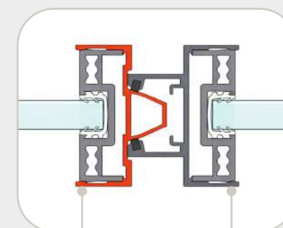
Смыкающиеся для синхро
