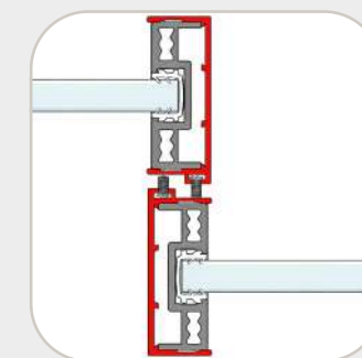
Межсекционные с щеточным уплотнителем
