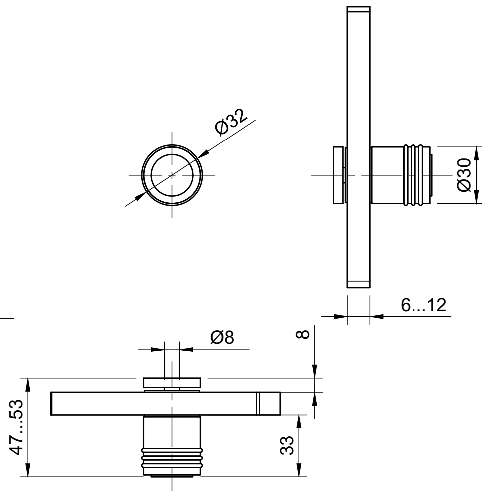
Эскиз установочных отверстий в стекле
