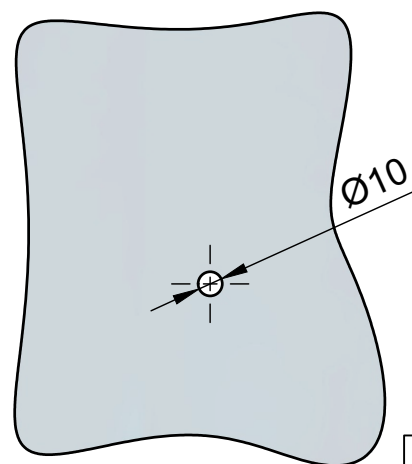
Эскиз установочных отверстий в стекле
