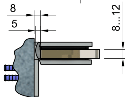
Отверстие в стекле с фиксирующими винтами
