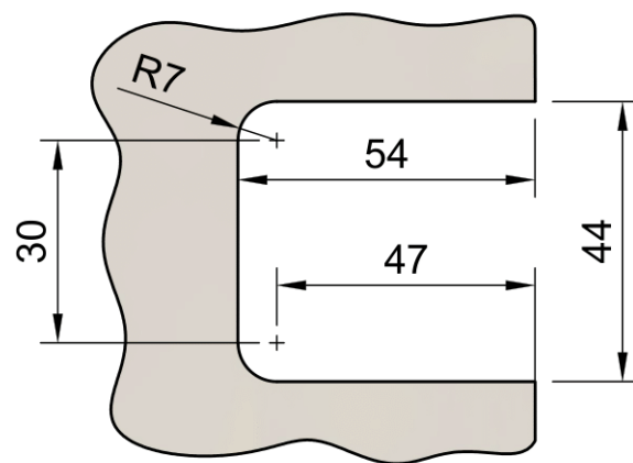
Отверстие в стекле без фиксирующих винтов
