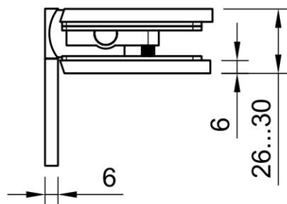
Отверстие в стекле без фиксирующих винтов
