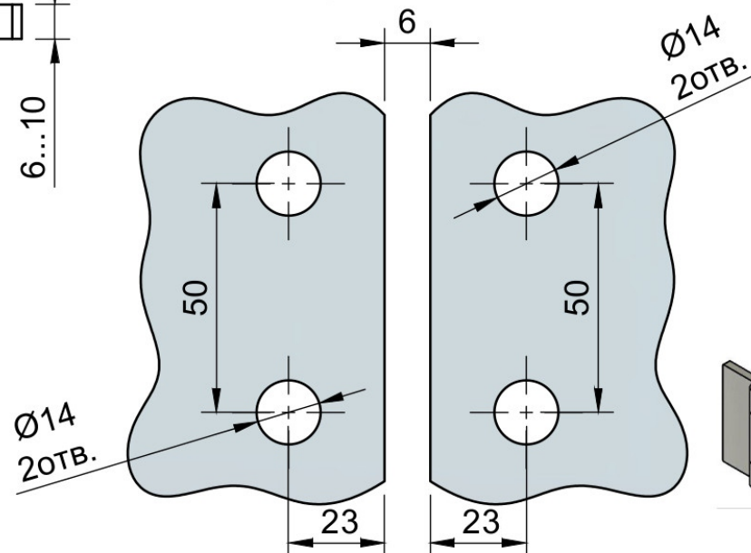
Эскиз установочных отверстий в стекле
